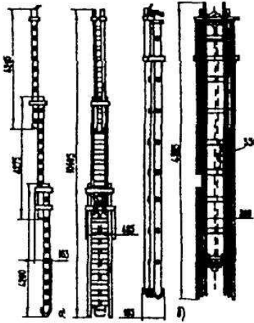
Рис. 5.1. Условное изображение приставной раздвижной лестницы Л-3К:
