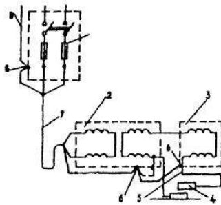
Рис. 7.1. Схема подключения сварочного трансформатора:
