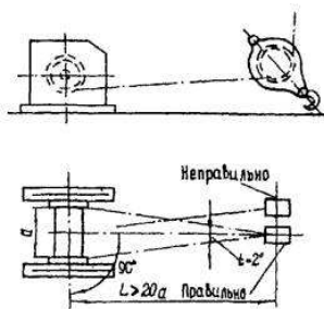
Рис. 4.2. Намотка каната на барабан лебедки
