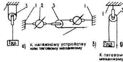
Рис. 4.3. Схема однорольных блоков:
