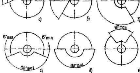
Рис. 3.1. Расположение и наибольшие допустимые углы раскрытия защитных кожухов:
