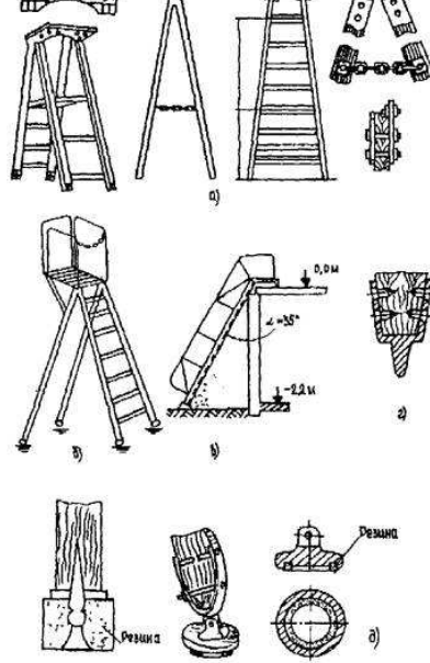
Рис. 5.3. Стремянки:
