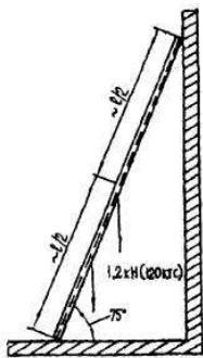
Рис. 5.5. Схема испытания приставной лестницы
