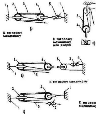
Рис. 4.4. Схема испытания многорольных блоков и полиспастов:
