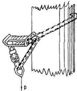
Рис. 6.1. Схема испытания монтерских когтей
