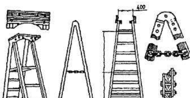
Рис. 5.2. Лестницы одноколенные:
