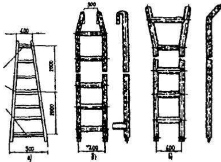
Рис. 5.2. Лестницы одноколенные:
